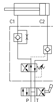
Esquema hidráulico Hydraulic diagram
