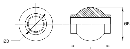
Bola para enganche rápido EPS y EPM (página 24). Ball for rapid hook EPS and EPM (page 24). Tratamiento zinc trivalente. Zinc trivalent treatment.
