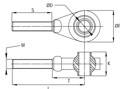
Rótula roscada para cilindro tercer punto Serie 600 (página 14). Ball for hydraulic top link 600 series (page 14). Tratamiento zinc trivalente. Zinc trivalent treatment.
