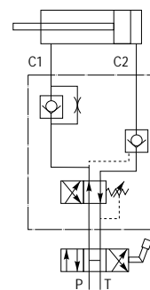
Esquema hidráulico válvula Hydraulic valve diagram
