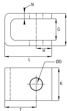
Material en S152.3 / Material in S152.3. Otras medidas bajo pedido / Other measures on request.
